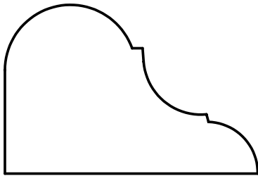
CM 144 11/16 X 1 3/8
